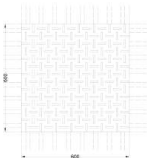
Disegno n. 5 – Codice di "Incrocio a "+" o a "T".
