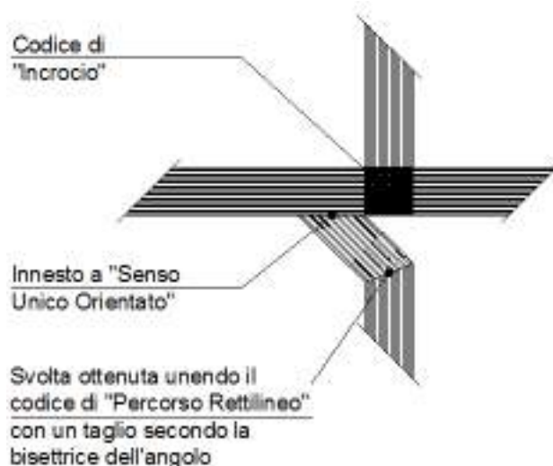
Disegno n. 11a – Percorso rettilineo a senso unico innestato in un segnale di INCROCIO.
